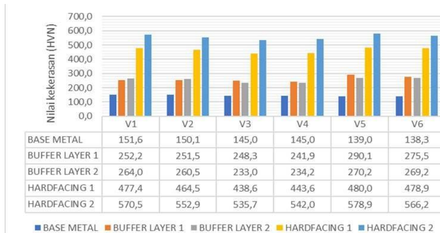
Fig. 3. Nilai kekerasan (HVN)
